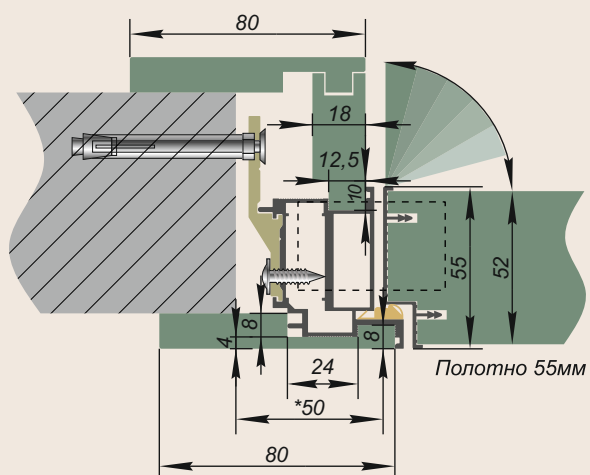
открывание в проём (IN)
