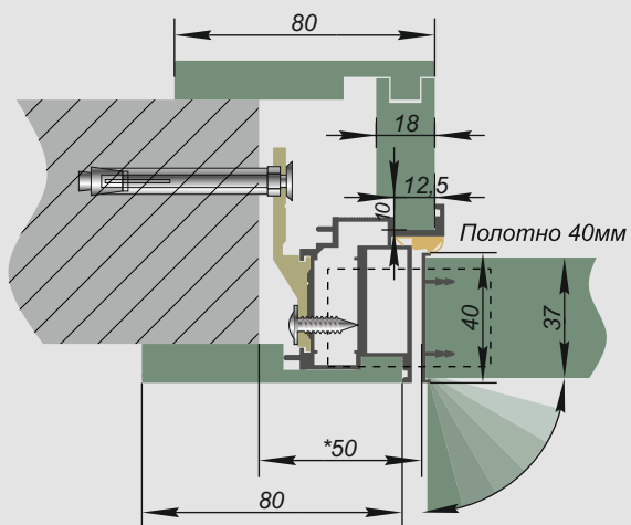
открывание из проёма (OUT)
