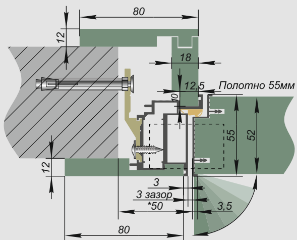
открывание из проёма (OUT)
