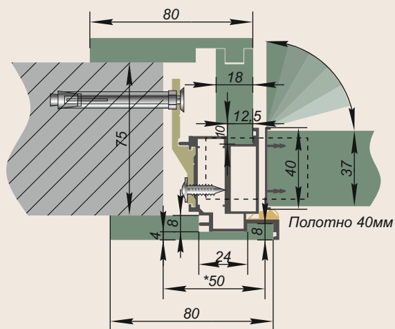
открывание в проём (IN)
